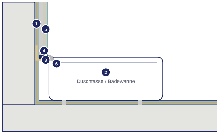
Anschluss Duschtasse/Badewanne an die Wand, Schnitt, schematisch, nicht maßstäblich.
